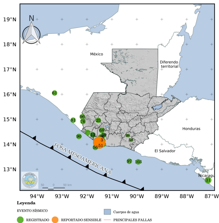
Figura 1: Localización geográfica de los 109 eventos sísmicos registrados en las últimas 24 horas
